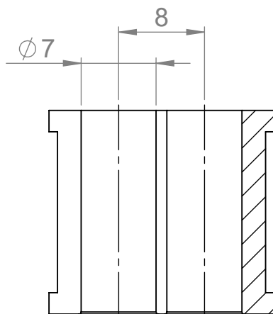
SCHNITT A-A
