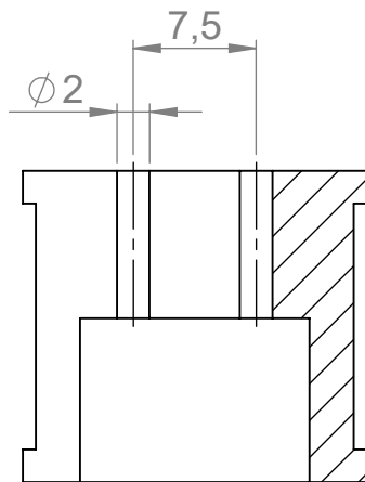
SCHNITT A-A
